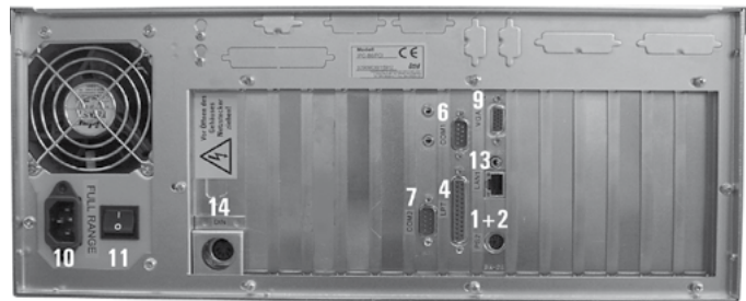
Bild: Anschlussfeld IPC-B mit Back- plane (Beispieldar- stellung, abhängig von den verwen- deten Hardware- komponenten und Bauteilen)
