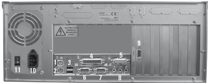
Bild: Anschlussfeld IPC-B mit ITX/ATX- Motherboard (Beispieldarstellung, abhängig vom verwendeten Motherboard)
