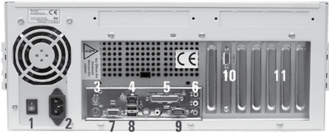
Bild: Anschlussfeld IPC-ECO mit ITX/ATX-Motherboard (Beispieldarstellung, abhängig von den verwendeten Motherboard)
