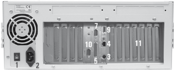
Bild: Anschlussfeld IPC-ECO mit Backplane (Beispieldarstellung, abhängig von den verwendeten Hardwarekomponenten und Bauteilen)
