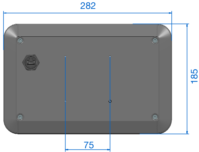
Unten / Bottom view
